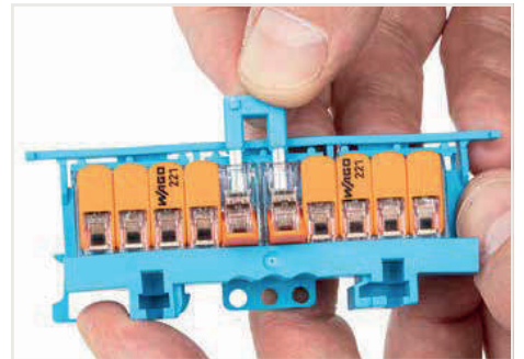
Köprüyü açık kelepçeleme birimlerinden çıkarın.
