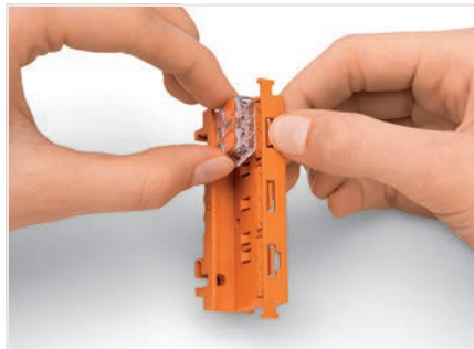
Bir konnektörü montaj taşıyıcısından çıkarma.
