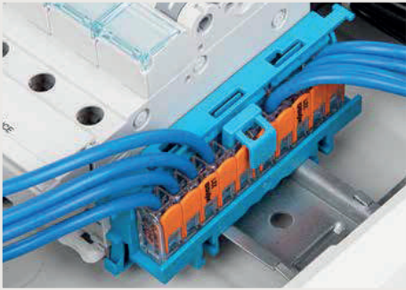
Kilitleme fonksiyonu ile: Kilitleme işlevine sahip köprü, ekleme konektörlerine takılır.
