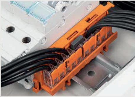
Kilitleme fonksiyonu olmadan: Kilitleme işlevi olmayan köprü, ekleme konektörlerine takılır.
