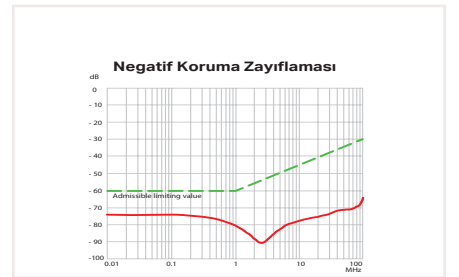
Blendaj bağlantı sistemi oldukça etkilidir çünkü sıkıştırma ünitesi kablunun blendajsız kısmına çok yaklaştırılabılır.
