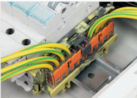
Kilitlelenebilir köprü, ekleme konektörlerine takılır.
