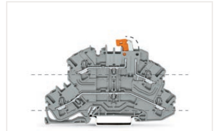
Bıçaklı ayrılmalı çift katlı ayırma klemensleri (2002-2671) Alt kattakiler geçiş klemensleri, üst kattakiler ayırma klemensleri olarak kullanılabilir.
